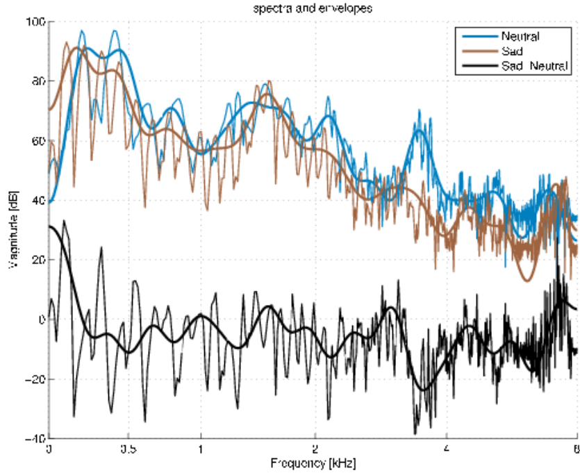
Figura 2: Involupi spettrali (linea spessa) e DFT (linea fine) di una coppia di frame coerenti (neutro e triste) e la loro differenza (triste-neutro). La scala delle ascisse è proporzionale alla scala mel.
