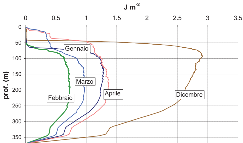
Fig. 2.6. Sequenza temporale della distribuzione verticale della stabilità termica del Lago Maggiore da Dicembre 2013 ad Aprile 2014.
