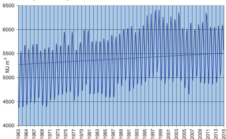
Fig. 2.2. Andamento mensile del contenuto di calore nella colonna d'acqua del Lago Maggiore nel periodo 1963-2014.
