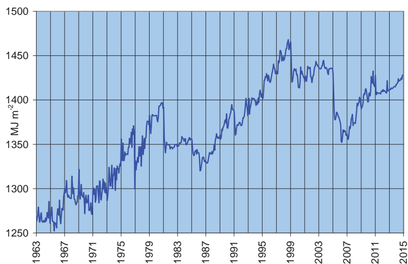
Fig. 2.3. Andamento della memoria climatica nel Lago Maggiore nel periodo 1963-2014.
