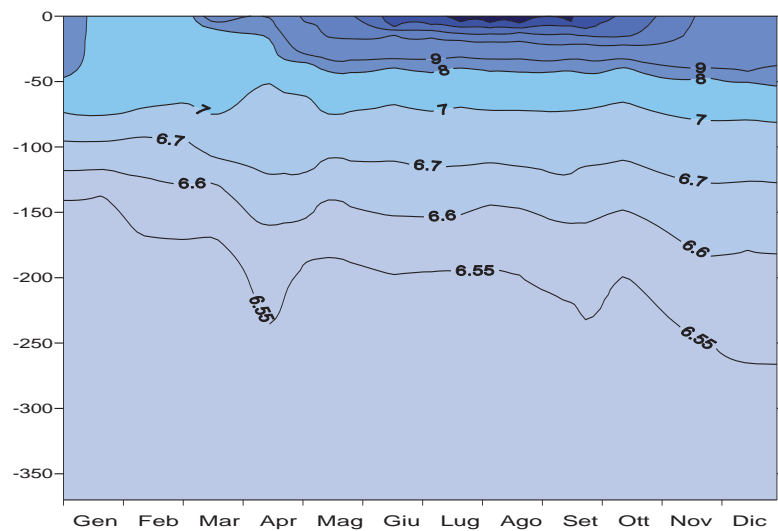
Fig. 2.5. Distribuzione verticale della temperatura (°C) nell'anno 2014.
