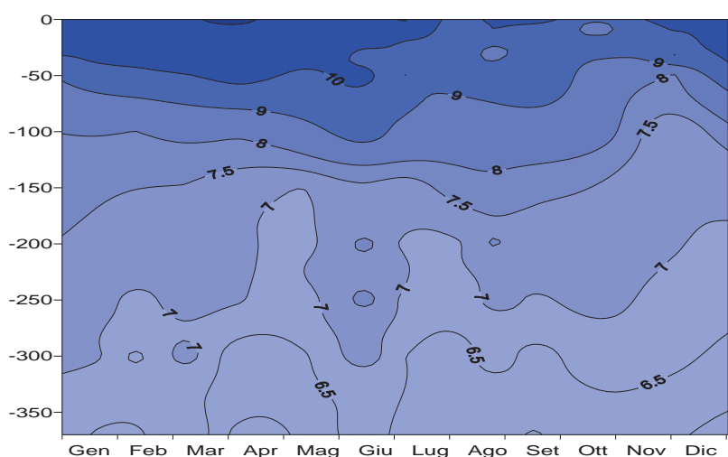
Fig. 2.4. Distribuzione verticale della concentrazione di O_2 ( \text{mg l}^{-1} ) nell'anno 2014.
