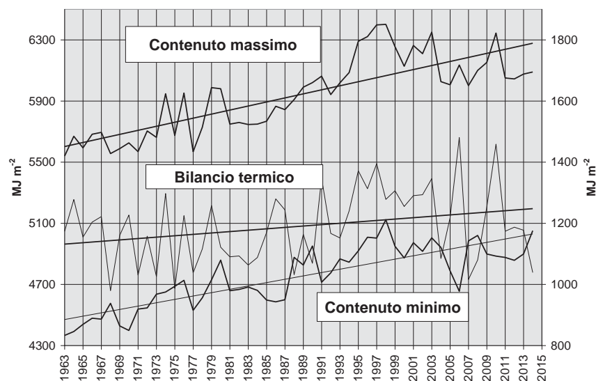
Fig.2.1. Contenuti di calore e bilancio termico delle acque del Lago Maggiore nel periodo 1963-2014.
