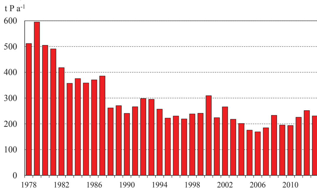
Fig. 7.18 Apporti annuali complessivi (areale emerso + zona rivierasca) di fosforo totale al Lago Maggiore nel periodo 1978-2013.
