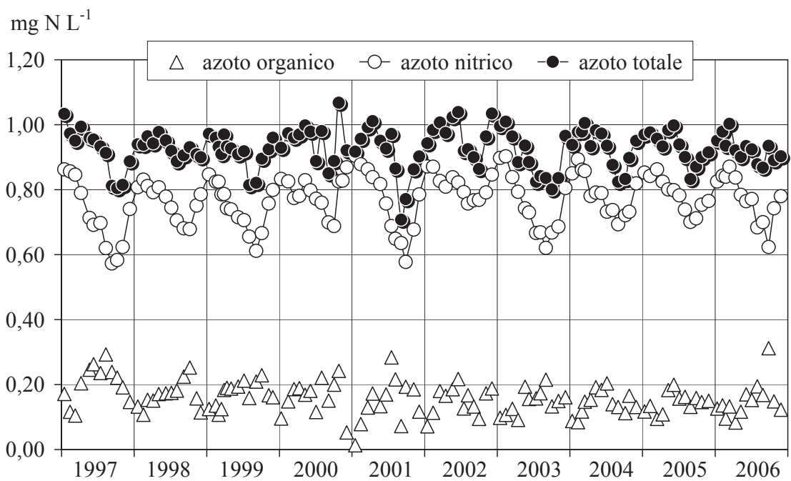
Fig. 3.2.2b. Concentrazioni di azoto nitrico, organico e totale nello strato epilimnico (0-25 m) nel decennio 1997-2006 (valori medi ponderati sui volumi nella stazione di massima profondità).
