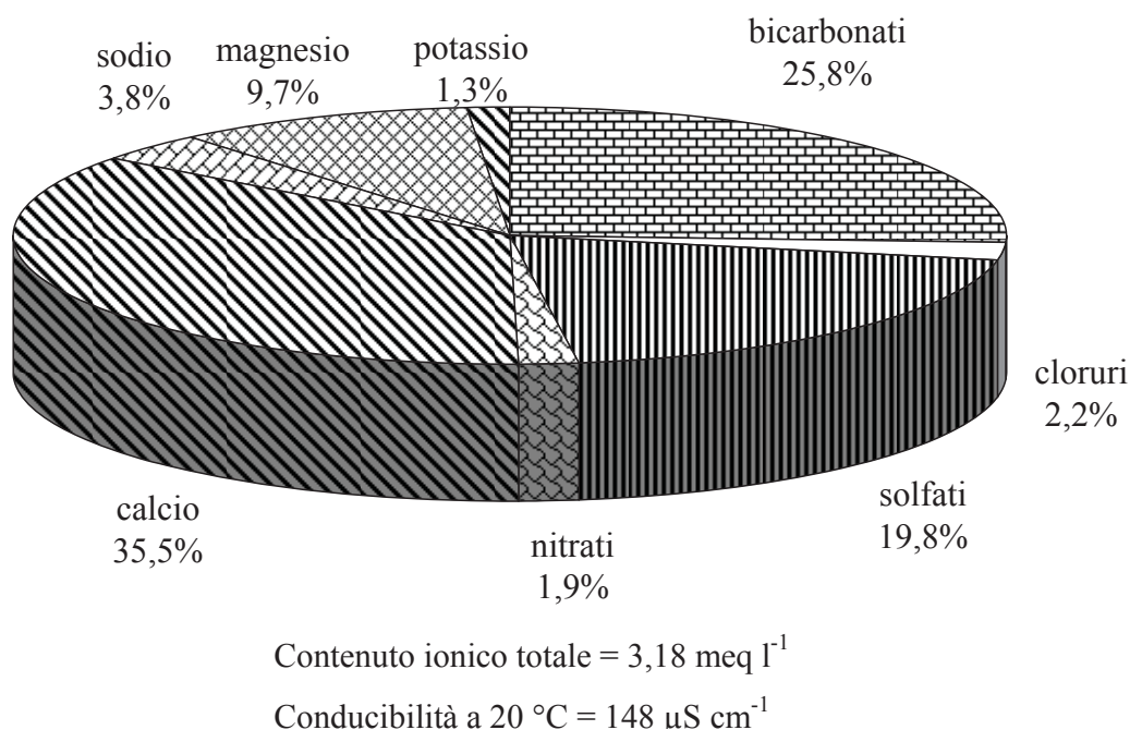
Fig. 3.2.1a. Lago Maggiore: ripartizione percentuale dello spettro ionico e valori medi di pH e conducibilità al 13 Marzo 2006 (valori medi ponderati sui volumi alla circolazione primaverile nella stazione di massima profondità).
