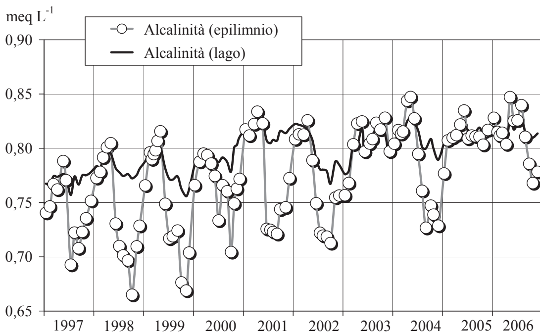
Fig. 3.2.1c. Lago Maggiore (Ghiffa). Andamento nel decennio 1997–2006 dei valori medi ponderati sui volumi d'alcalinità totale nello strato epilimnico (0-25 m) e nell'intero lago (0-370 m).
