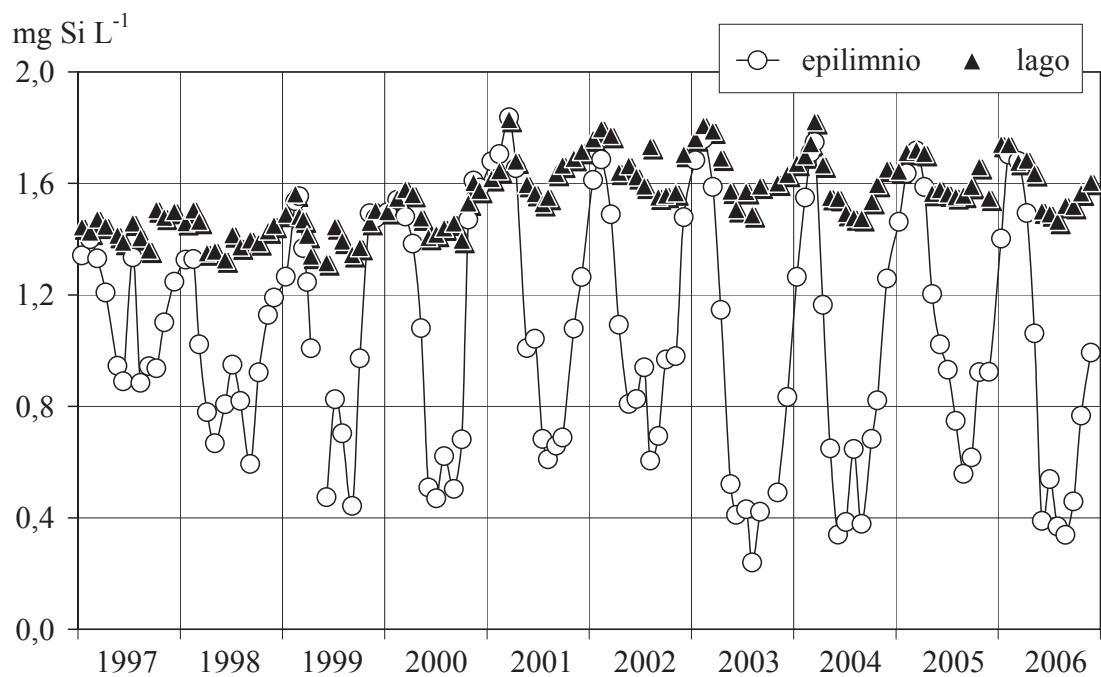
Fig. 3.2.5. Lago Maggiore (Ghiffa). Concentrazioni medie ponderate sui volumi di silicati reattivi nello strato epilimnico (0-25 m) e nell'intero lago (0-370 m) nel decennio 1997-2006.
