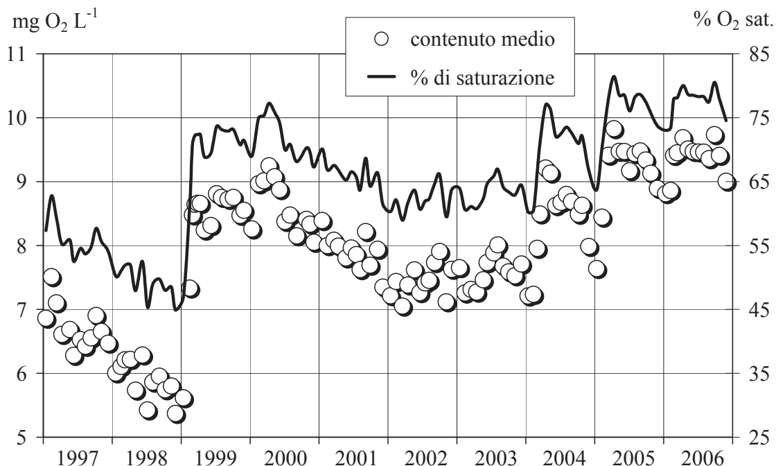
Fig. 3.2.4a. Lago Maggiore, stazione di Ghiffa. Andamento nel decennio 1997-2006 delle concentrazioni medie di ossigeno (valori ponderati sui volumi) e dei corrispondenti tenori di saturazione nello strato 200-370 m.
