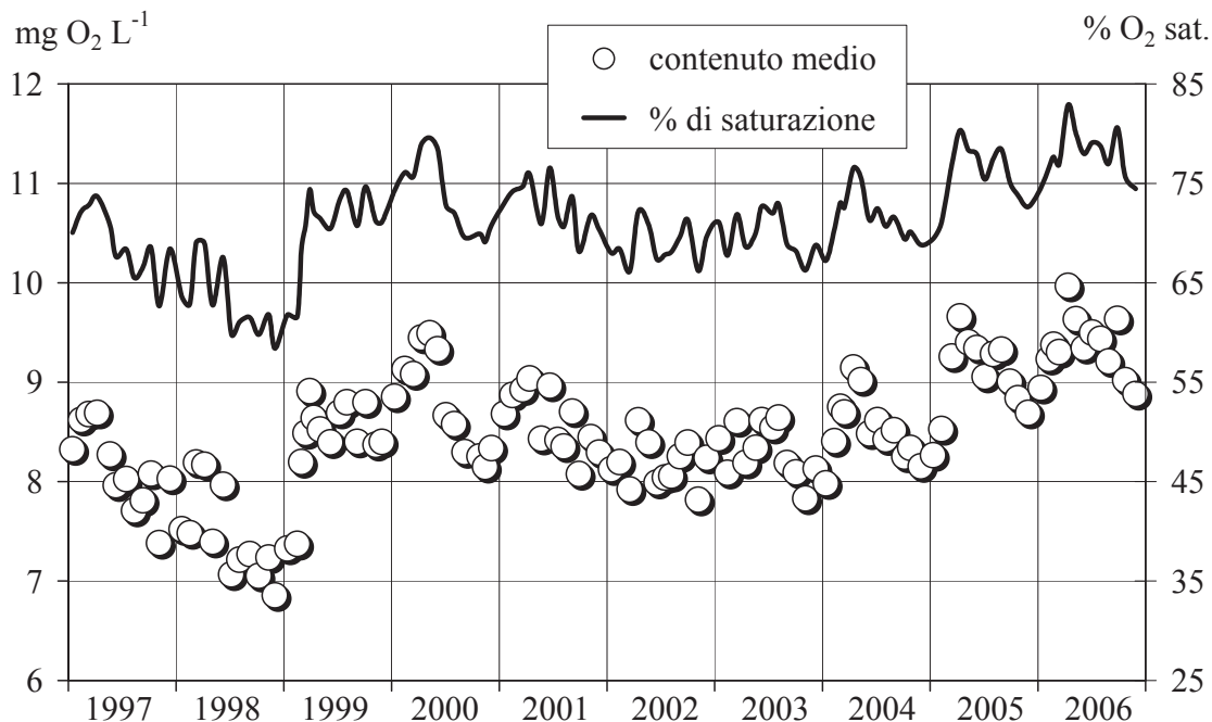
Fig. 3.2.4b. Lago Maggiore, stazione di Ghiffa. Andamento nel decennio 1997-2006 delle concentrazioni medie di ossigeno (valori ponderati sui volumi) e dei corrispondenti tenori di saturazione nello strato 25-370 m.
