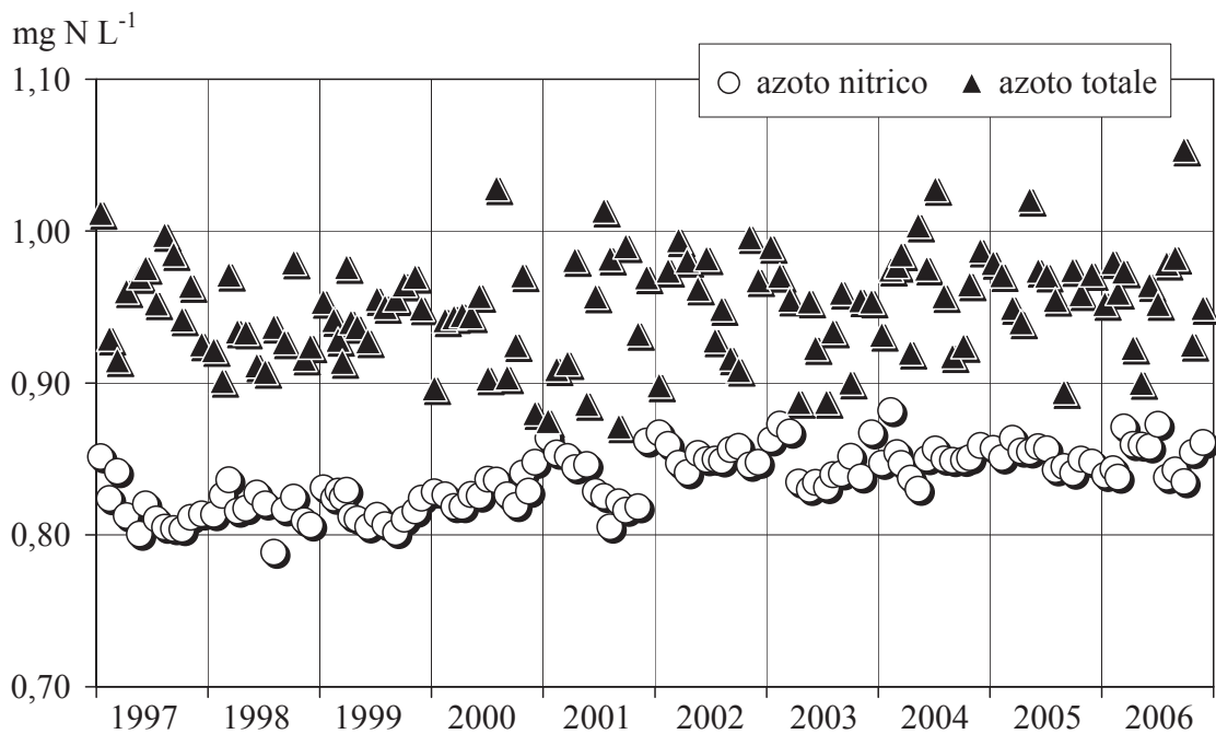
Fig. 3.2.2a. Lago Maggiore: concentrazioni di azoto totale e nitrico nel decennio 1997-2006 (valori medi ponderati sui volumi dalla superficie al fondo nella stazione di massima profondità).
