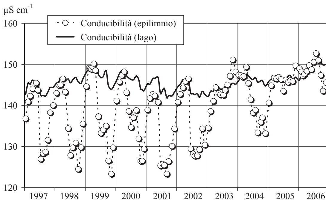
Fig. 3.2.1d. Lago Maggiore (Ghiffa). Andamento nel decennio 1997–2006 dei valori medi ponderati sui volumi di conducibilità a 20°C nello strato epilimnico (0-25 m) e nell'intero lago (0-370 m).
