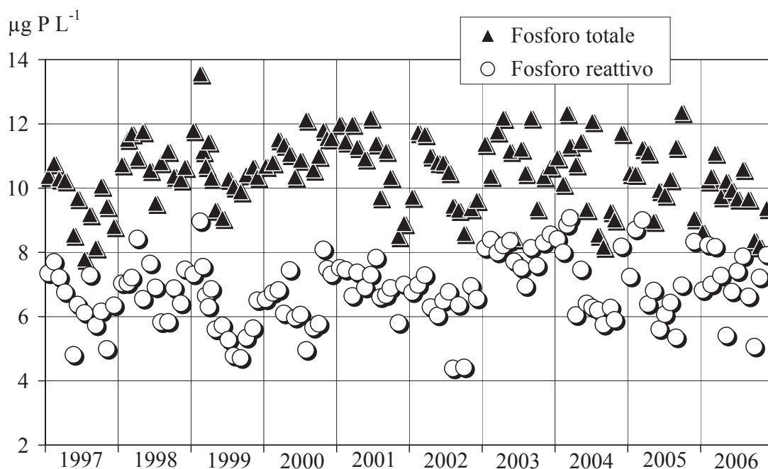
Fig. 3.2.3. Lago Maggiore: andamento delle concentrazioni di fosforo reattivo e totale nel decennio 1997-2006 (valori medi ponderati sui volumi dalla superficie al fondo nella stazione di massima profondità).
