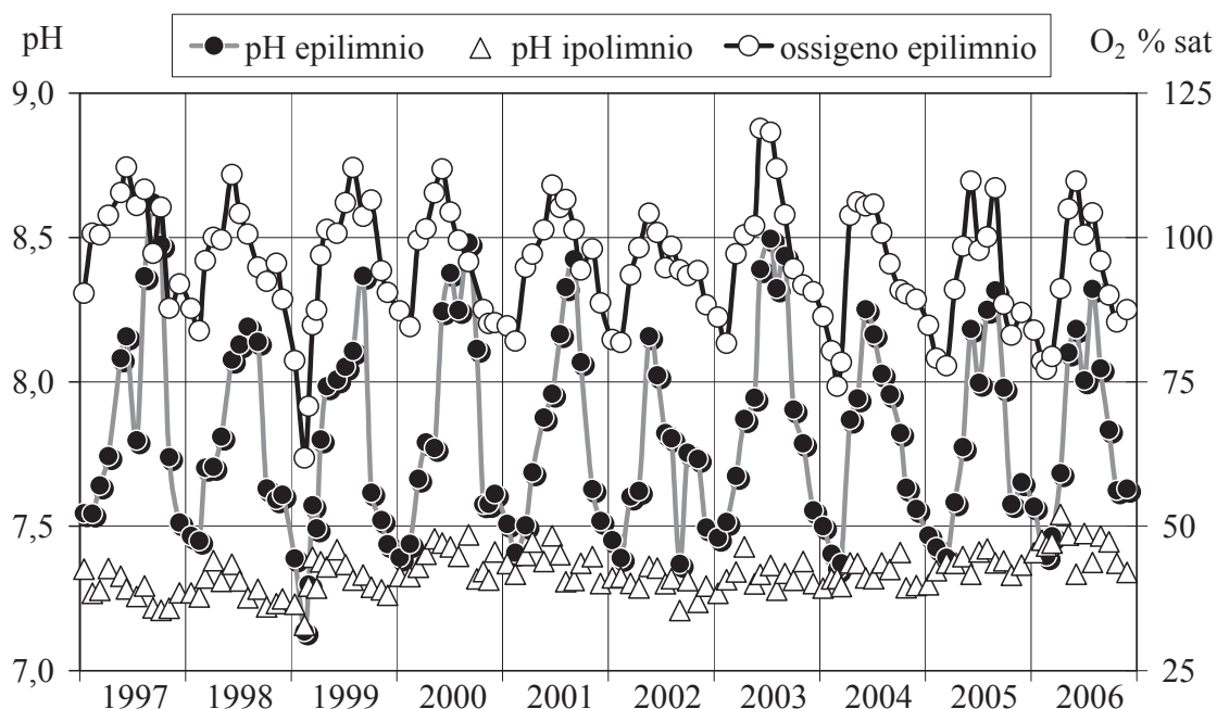
Fig. 3.2.1b. Lago Maggiore nel periodo 1997-2006: pH nello strato epilimnico (0-25 m) ed ipolimnico (25-370 m) e saturazione d'ossigeno nello strato epilimnico (valori medi ponderati sui volumi nella stazione di massima profondità).
